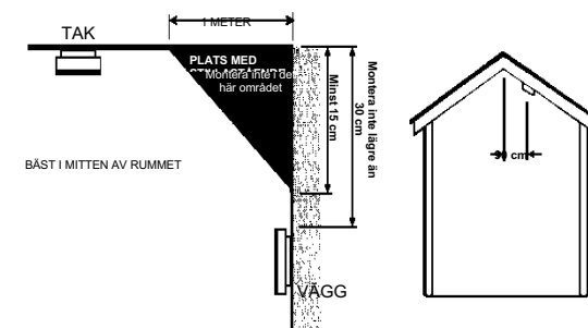
Figur 3i – Placering av brandvarnare
